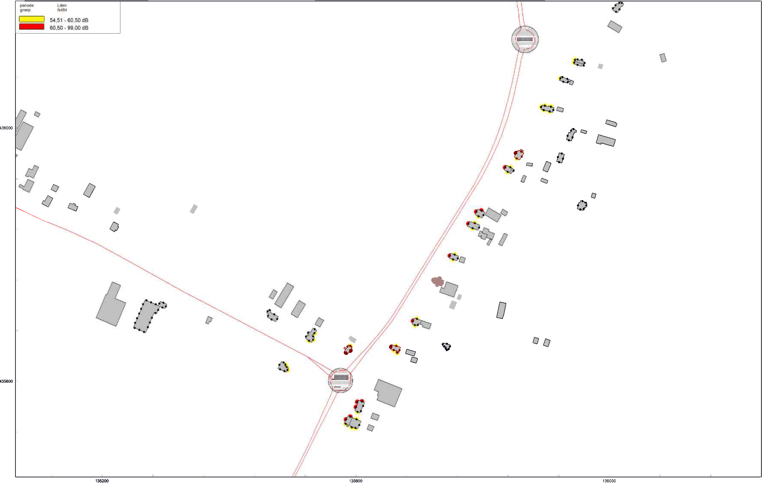
Figuur 2 | Woningen met plandrempel van > 61 dB en > 55 dB
