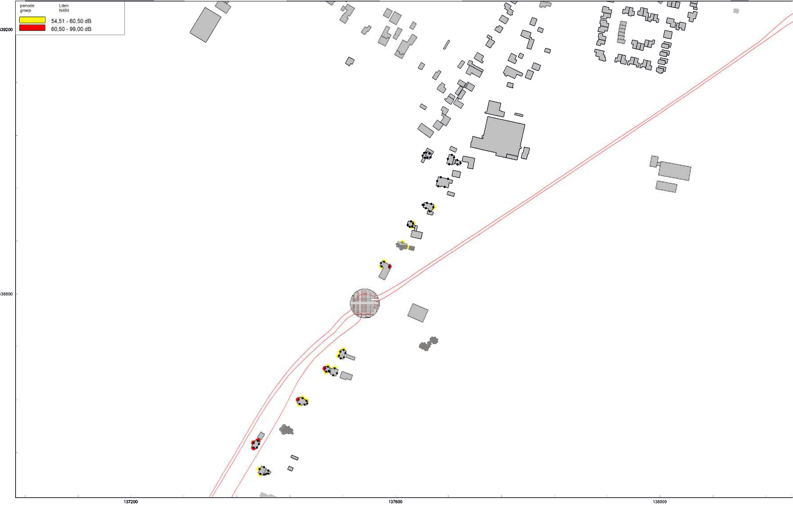
Figuur 7 | Woningen met plandrempel van > 61 dB en > 55 dB
