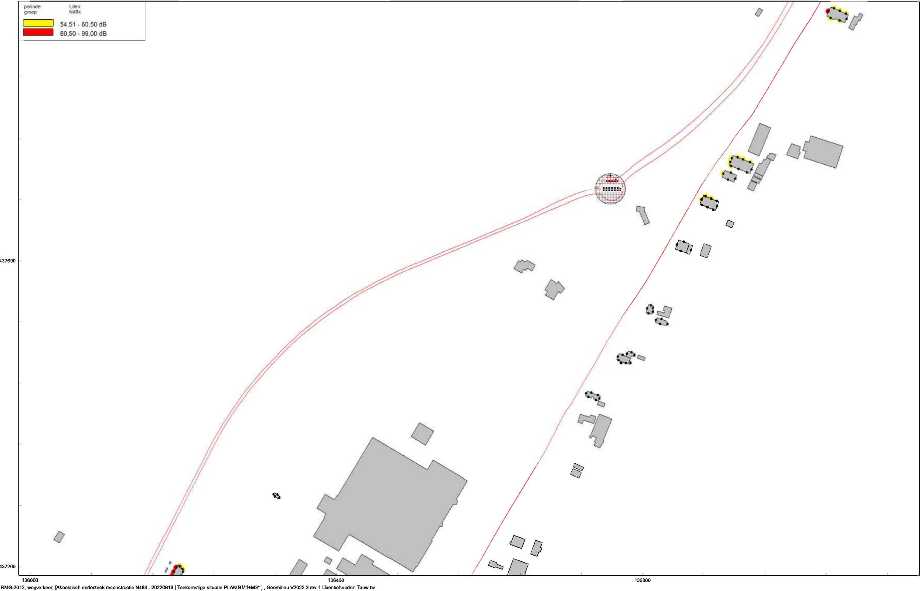
Figuur 5 | Woningen met plandrempel van > 61 dB en > 55 dB
