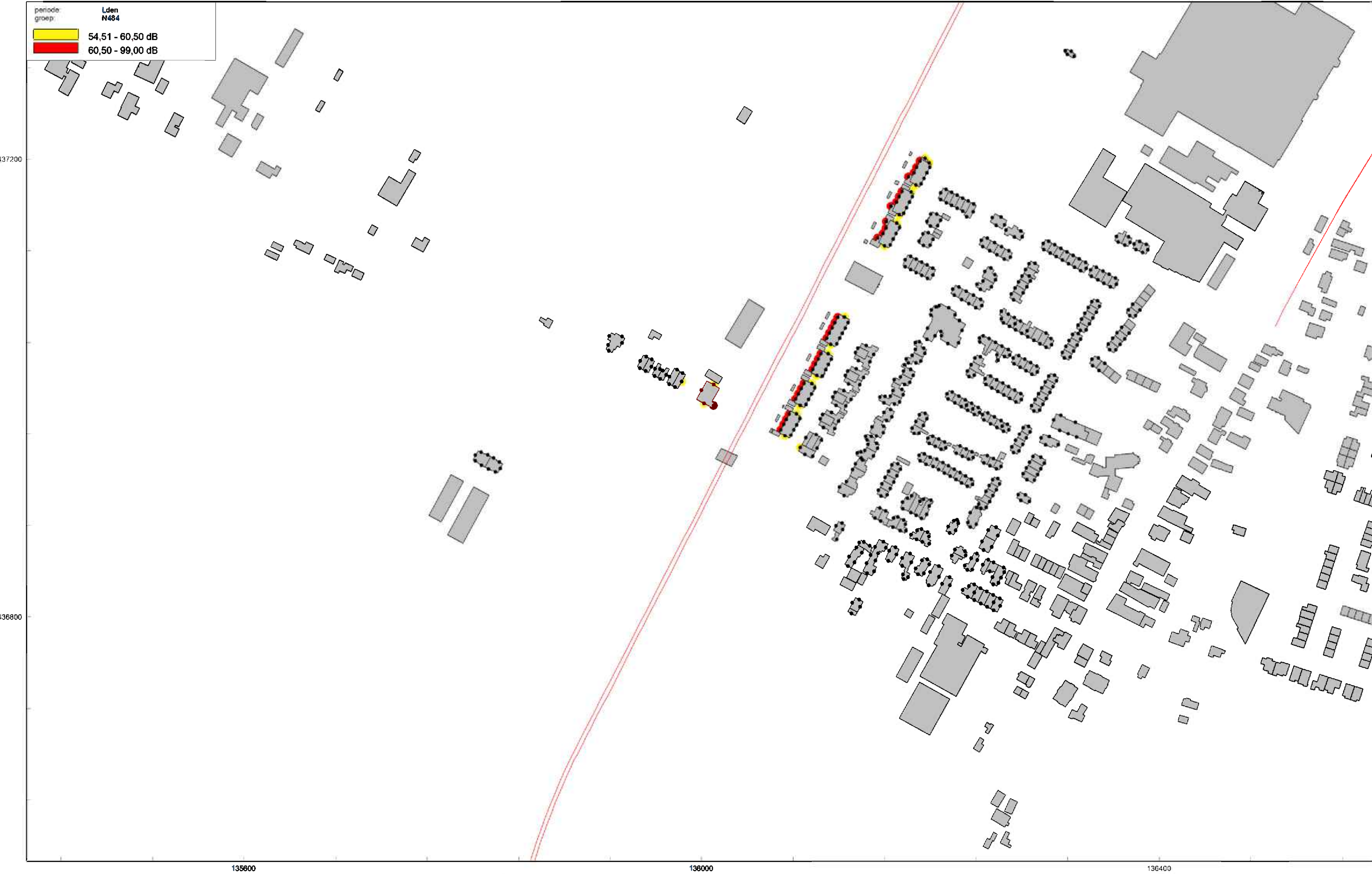
Figuur 4 | Woningen met plandrempel van > 61 dB en > 55 dB
