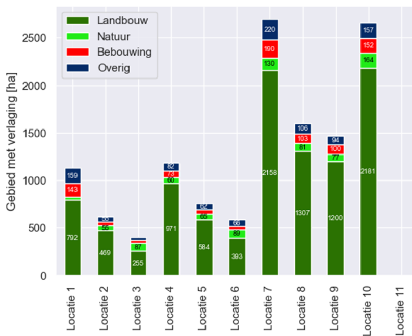
Afbeelding 4.3 Overzicht gebieden met aantal hectare verlaging per locatie
