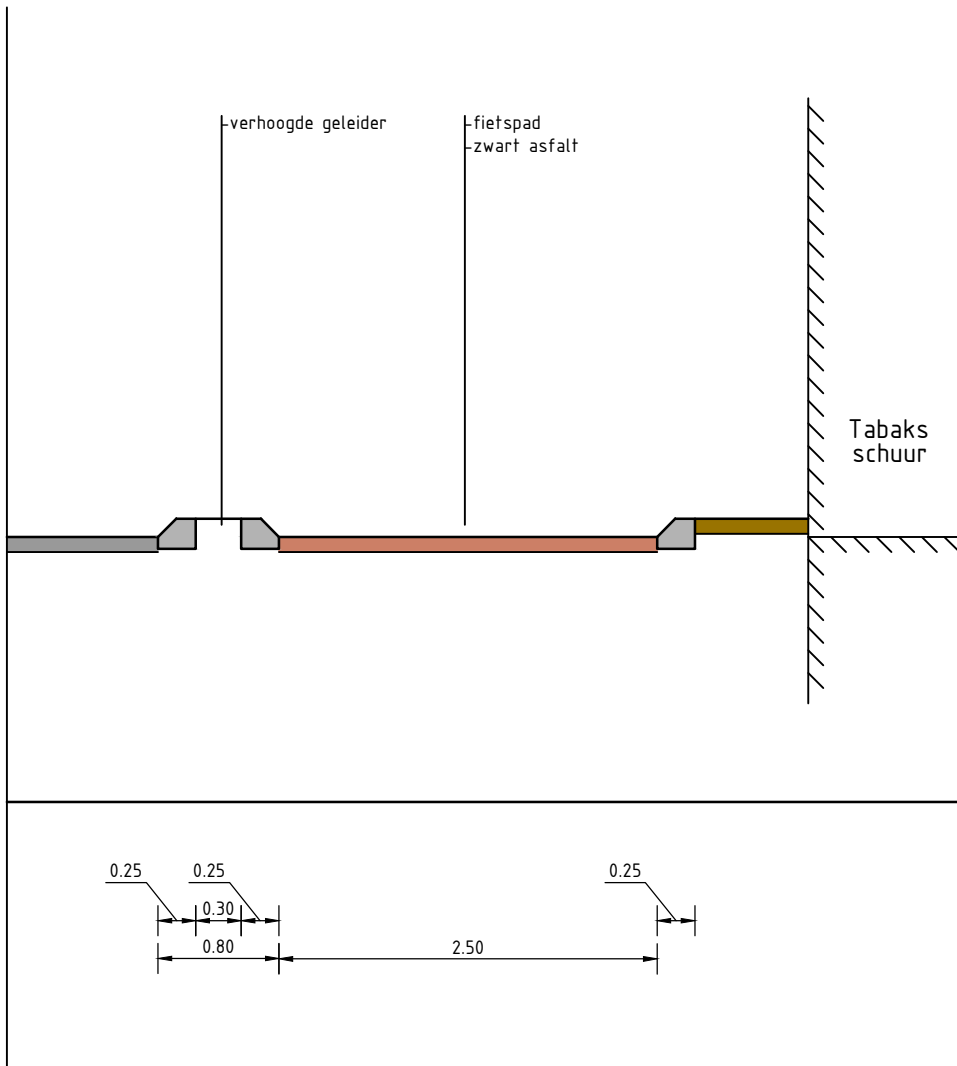
Doorsnede Bestaande situatie met RWS-banden Schaal 1:50
