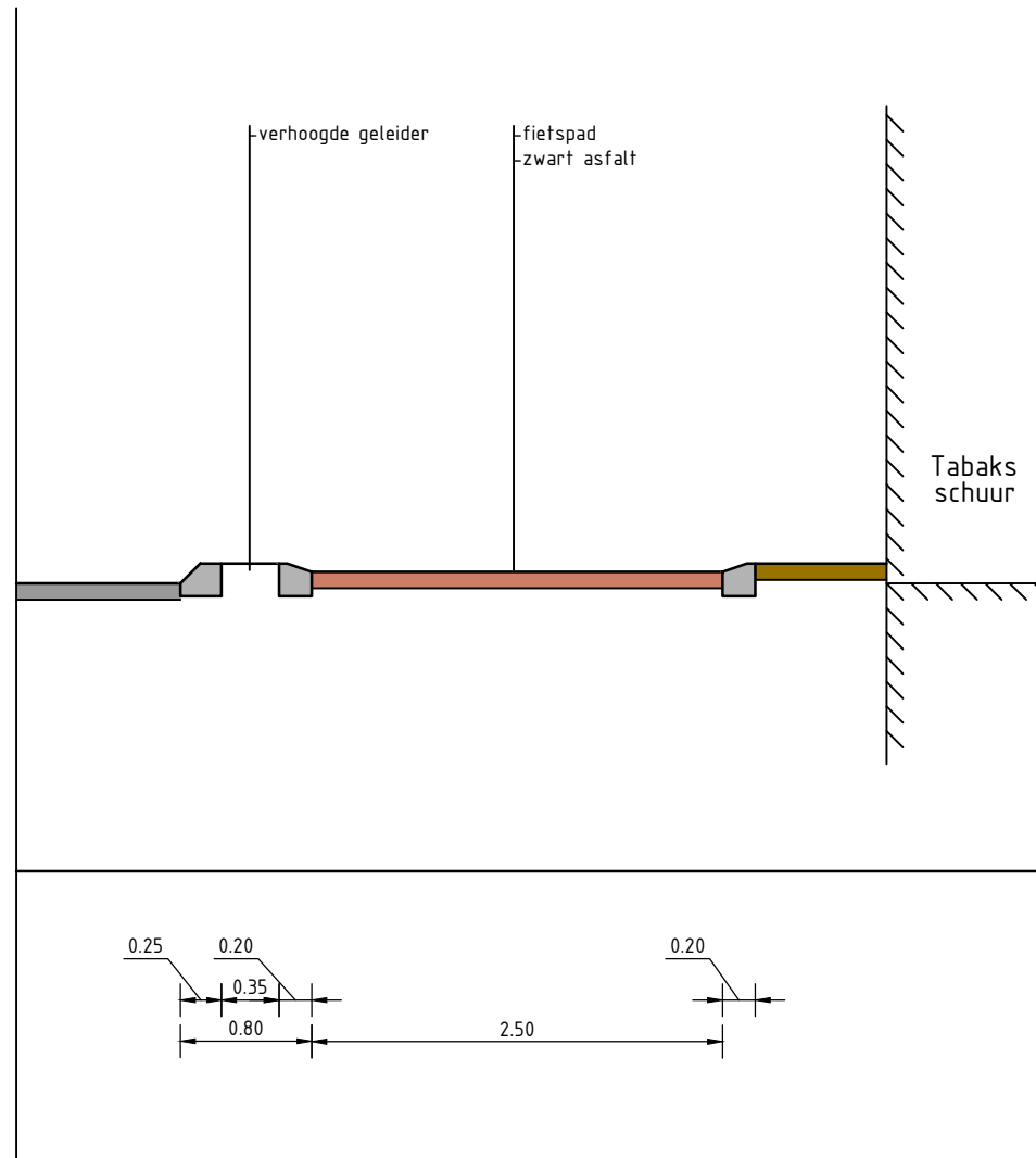
Doorsnede nieuwe situatie met RWS en geleidebanden Schaal 1:50
