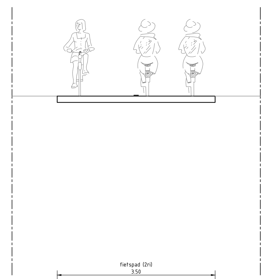
Doorsnede G-G Schaal 150
