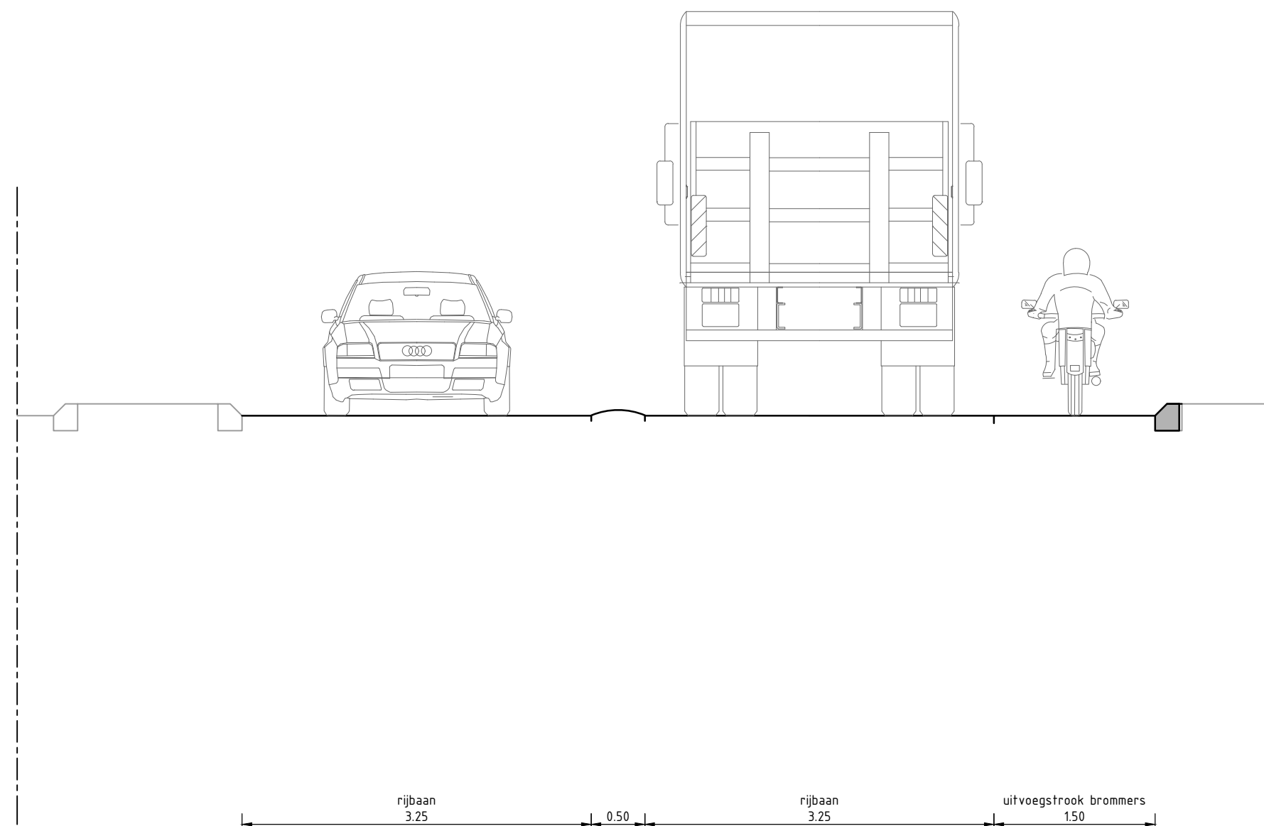
Doorsnede A-A Schaal 150
