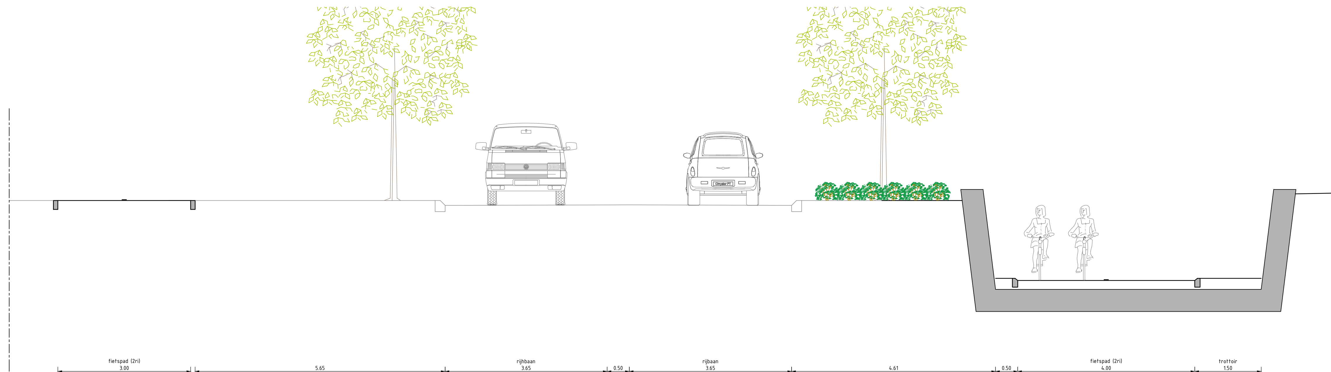
Doorsnede C-C Schaal 150
