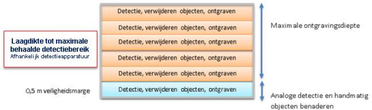
Figuur 40: Schematische weergave werkmethode laagsgewijze oppervlakedetectie
