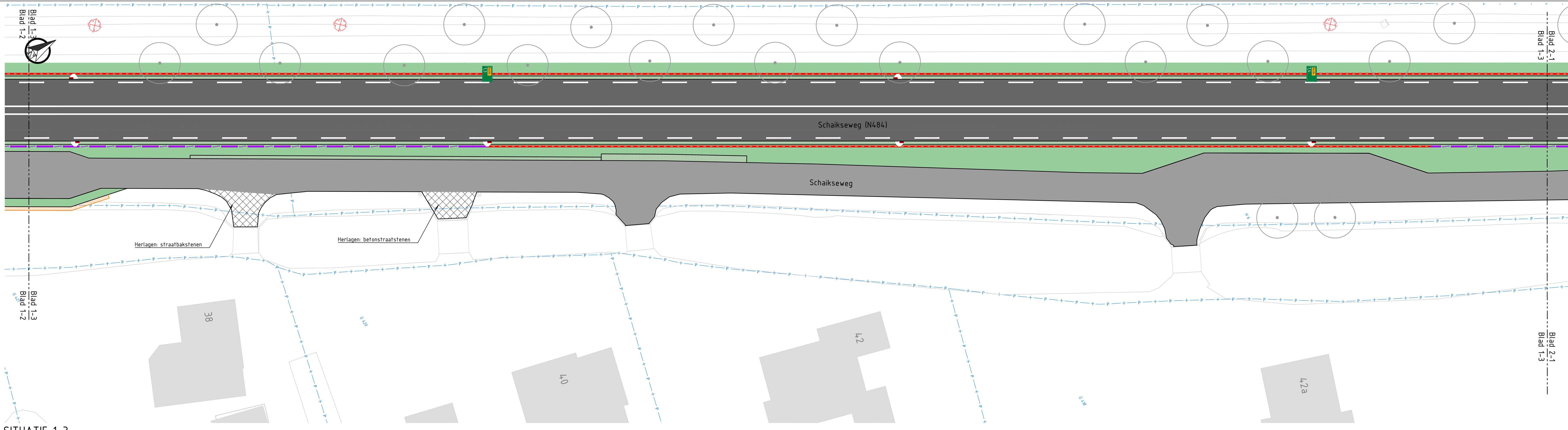
SITUATIE 1-3 SCHAAL 1 : 200
