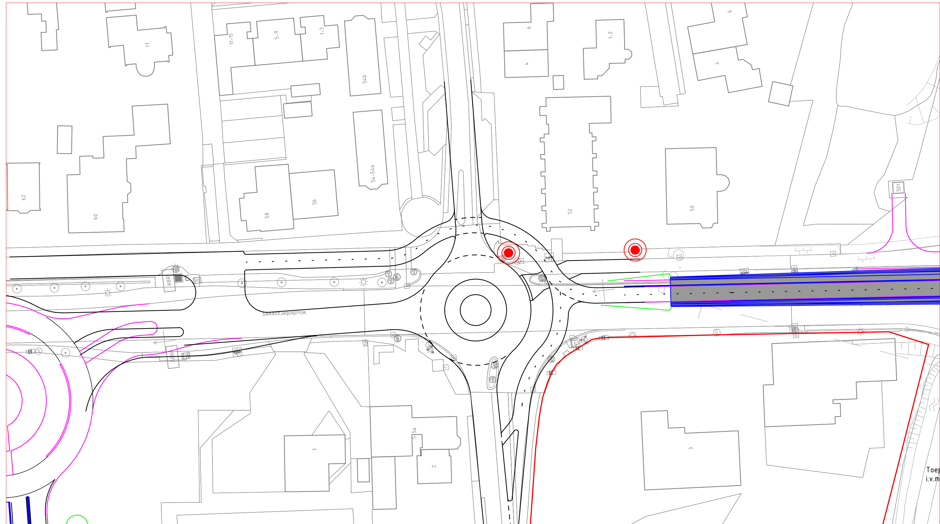
Variant III 'Rotonde, fietsers voorrang'
