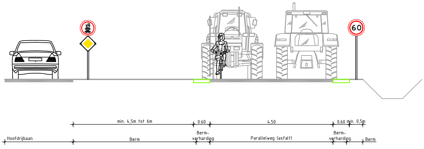
Profiel o.b.v. Handboek wegontwerp
