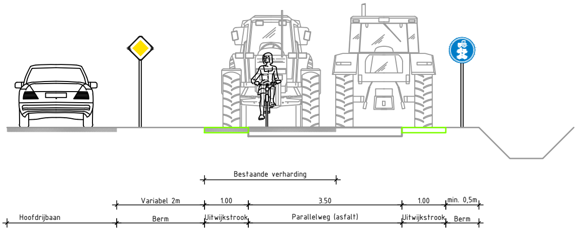
Profiel Alternatieve bebording
