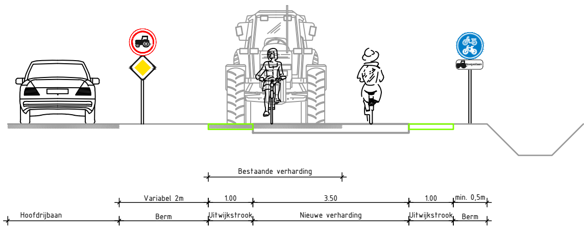
Profiel o.b.v. praktische inpassing
