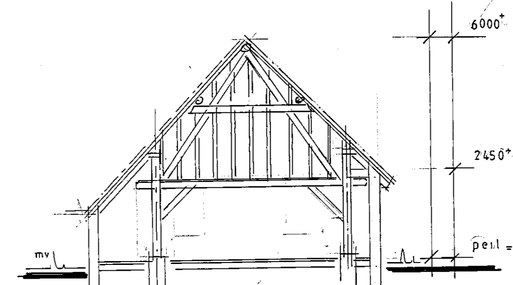
doorsnede
