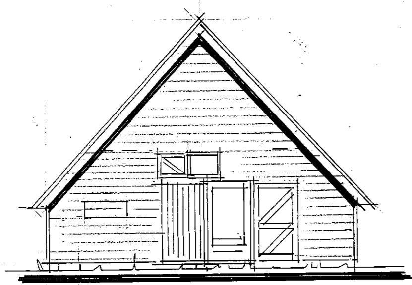
voorgevel
