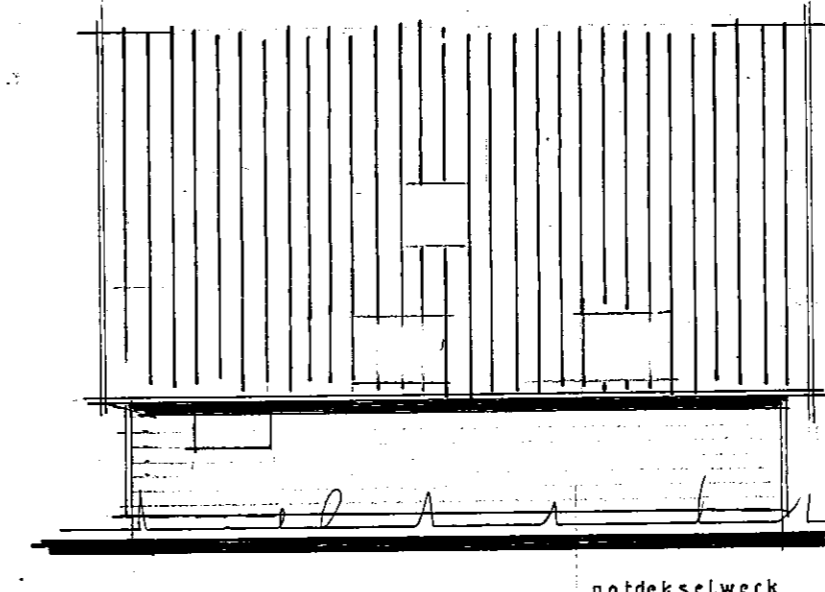
rechter zijgevel
