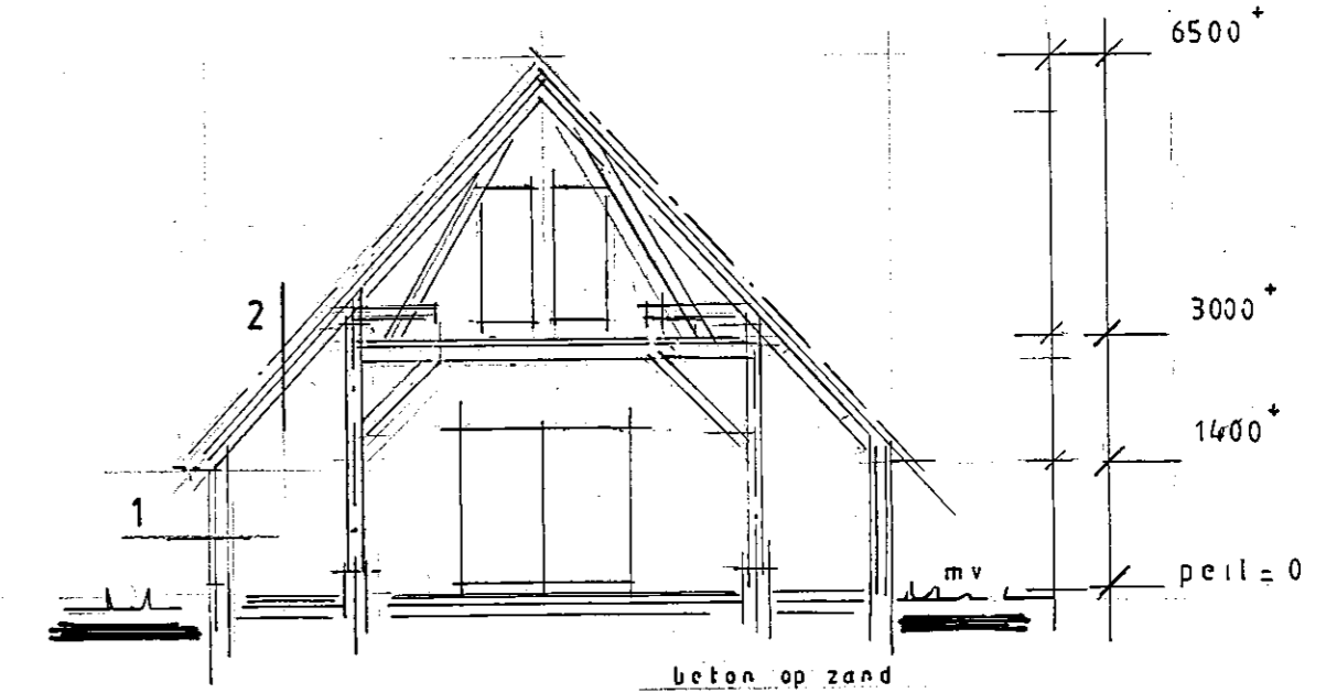
doorsnede
